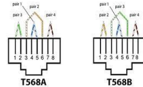
Wiring for T568B & T568A
